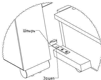
Схема тахты в положение «лежа»
